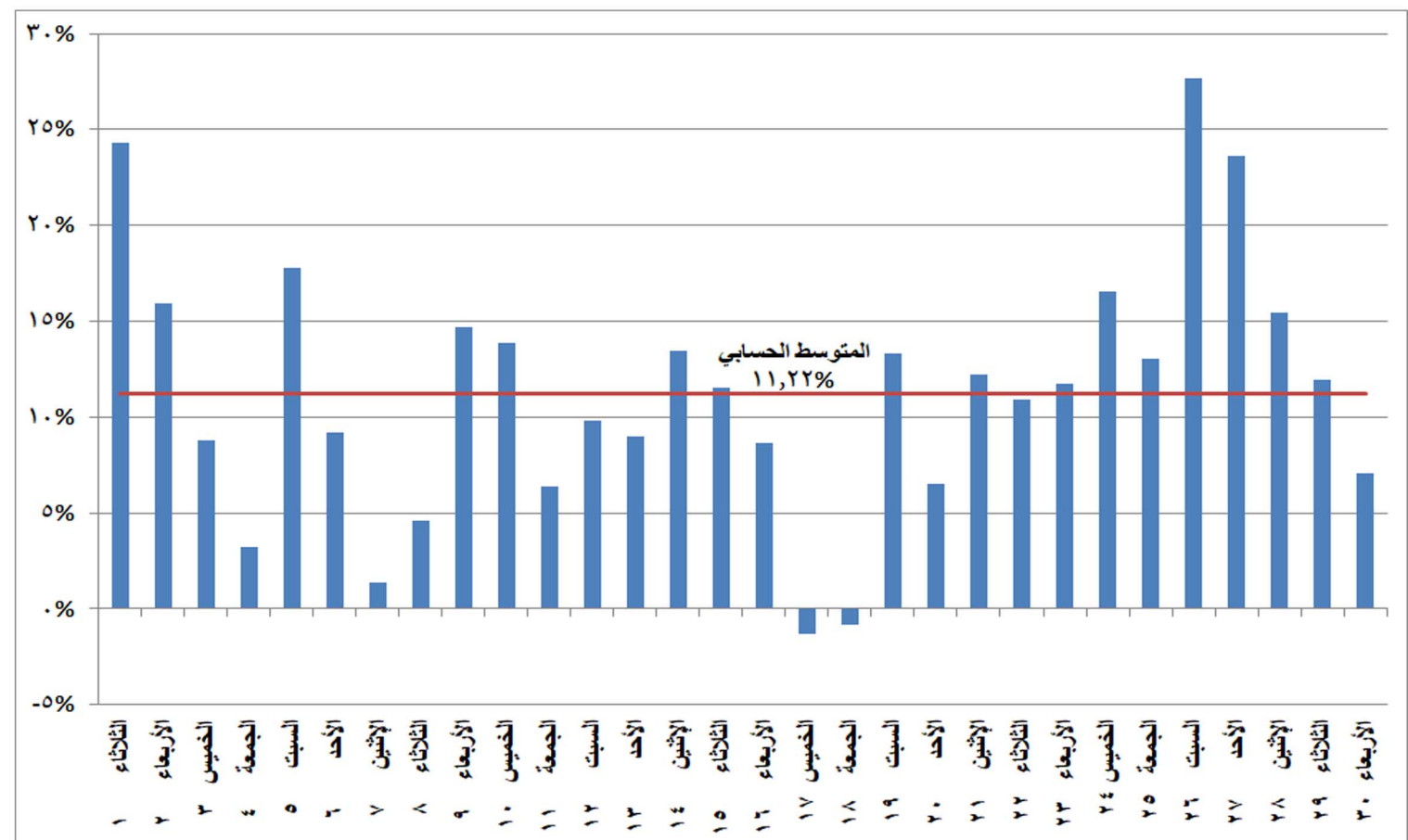
شكل (١٨) نسب التغير في استخدام الغاز الطبيعي في إنتاج الطاقة الكهربائية خلال شهر يونيو ٢٠٢١ مقارنة بالشهر المماثل من العام السابق
