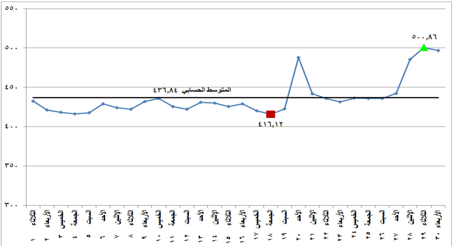
شكل (١٤) معامل انبعاثات غاز ثاني اكسيد الكربون المكافئ على مدى شهر يونيو ٢٠٢١
