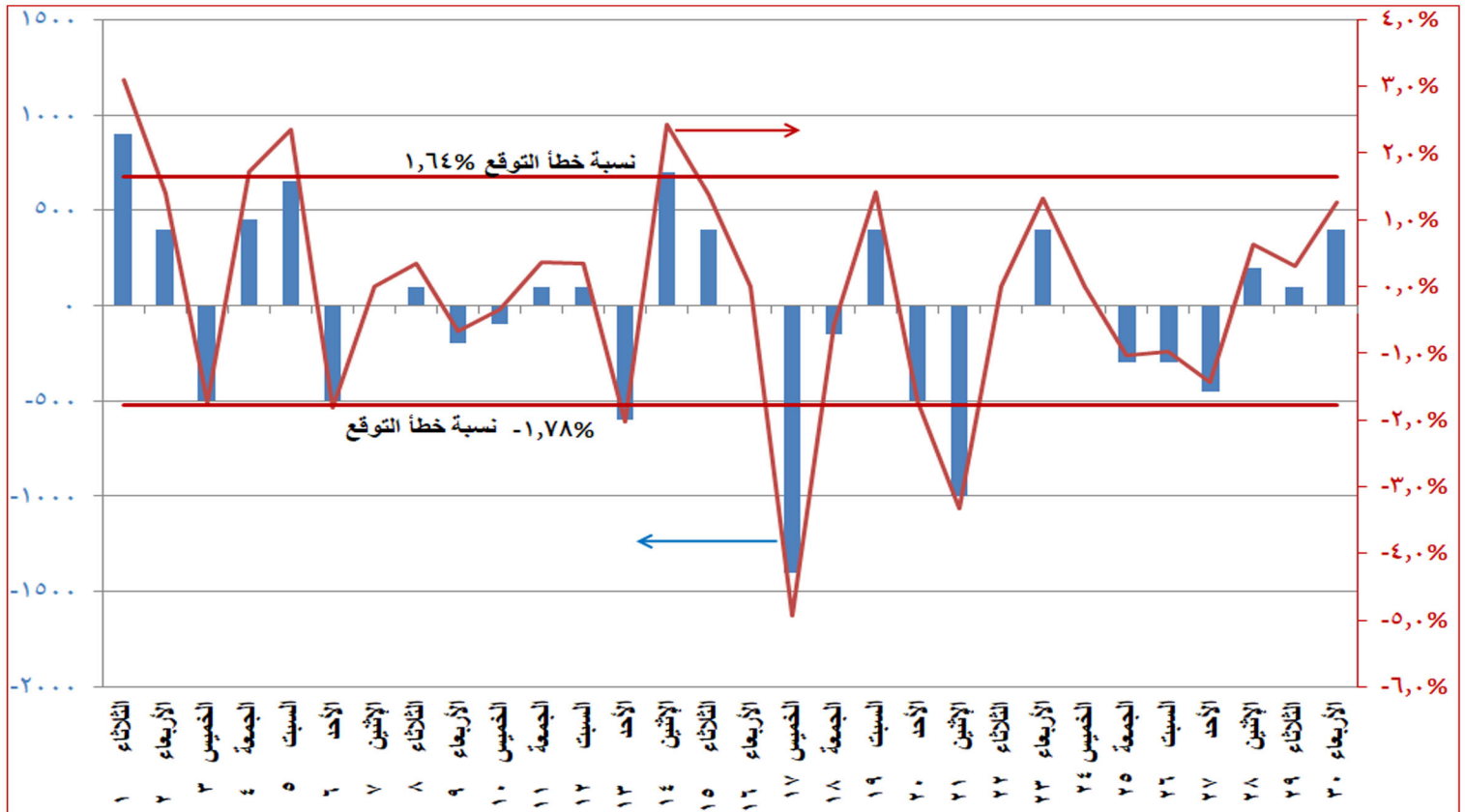
شكل (١٠) الفرق بين الحمل الأقصى المتوقع والمسجل فعليا ونسبة الفرق الى الحمل المسجل فعليا خلال شهر يونيو ٢٠٢١
