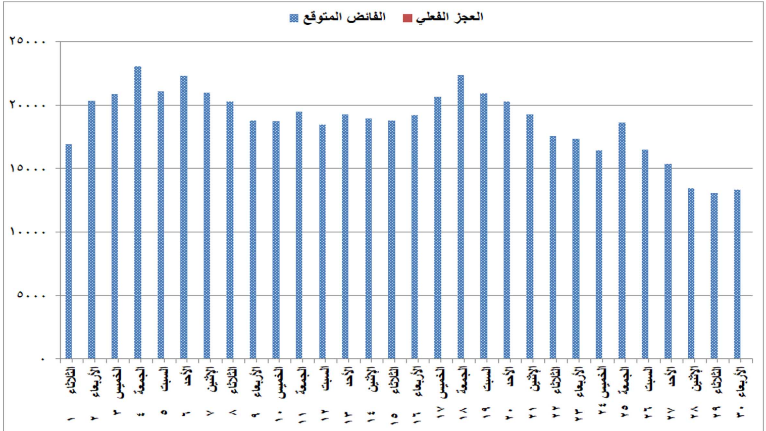
شكل (٧) الفائض والعجز المتوقع للقدرات خلال شهر يونيو ٢٠٢١
