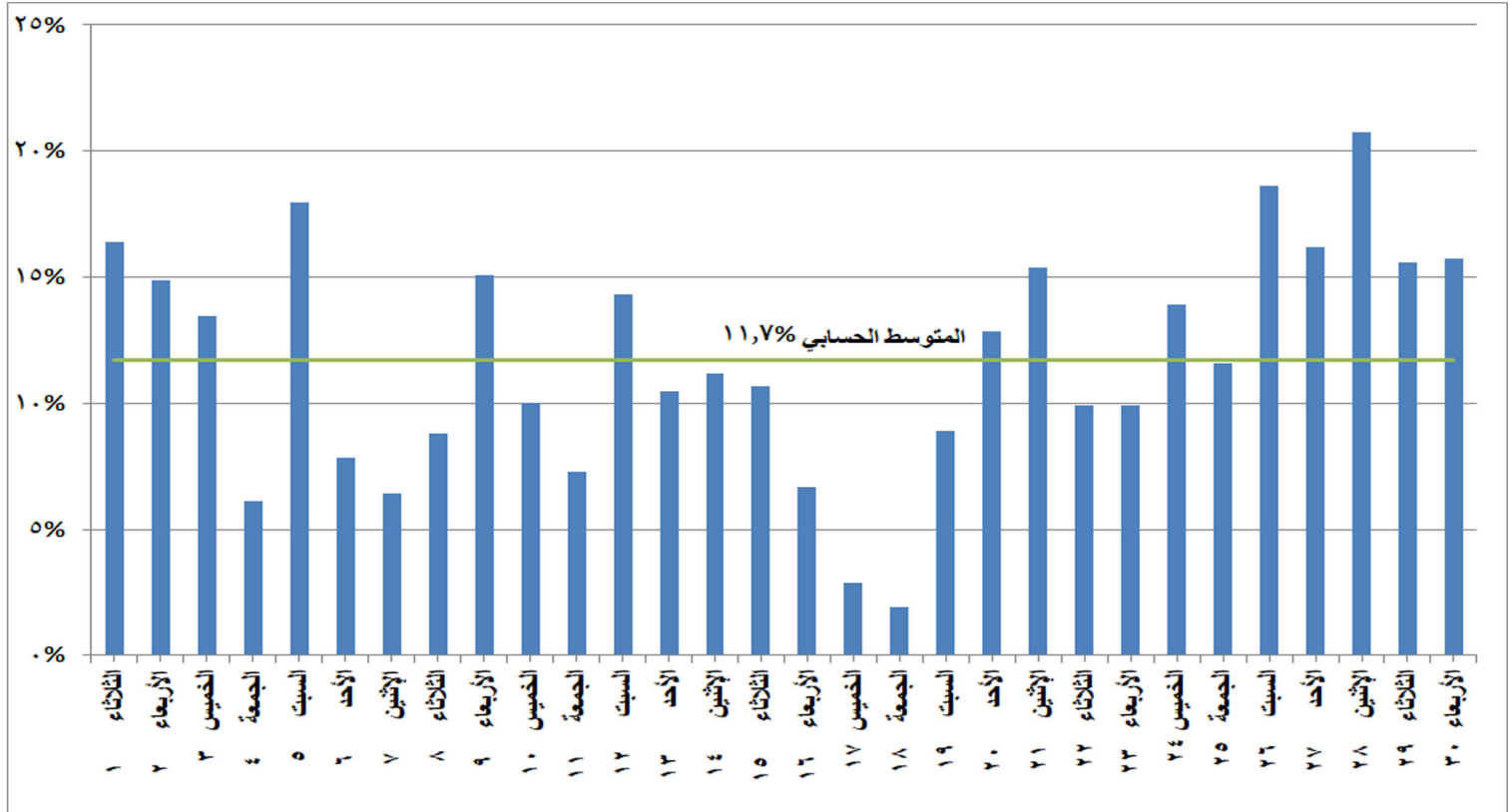
شكل (٩) النسب المئوية للتغير في الحمل الاقصى خلال شهر يونيو ٢٠٢١ مقارنة باليوم المماثل من العام الماضي
