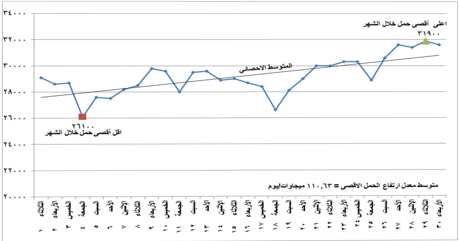
شكل (١) تطور الحمل الاقصى اليومي خلال شهر يونيو ٢٠٢١
