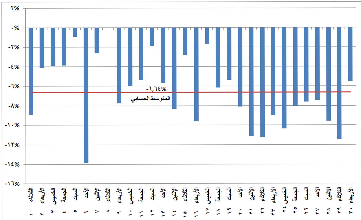
شكل (٢٤) نسب التغير في استخدام المصادر المائية في إنتاج الطاقة الكهربائية خلال شهر يونيو ٢٠٢١ مقارنة بالشهر المماثل من العام السابق
