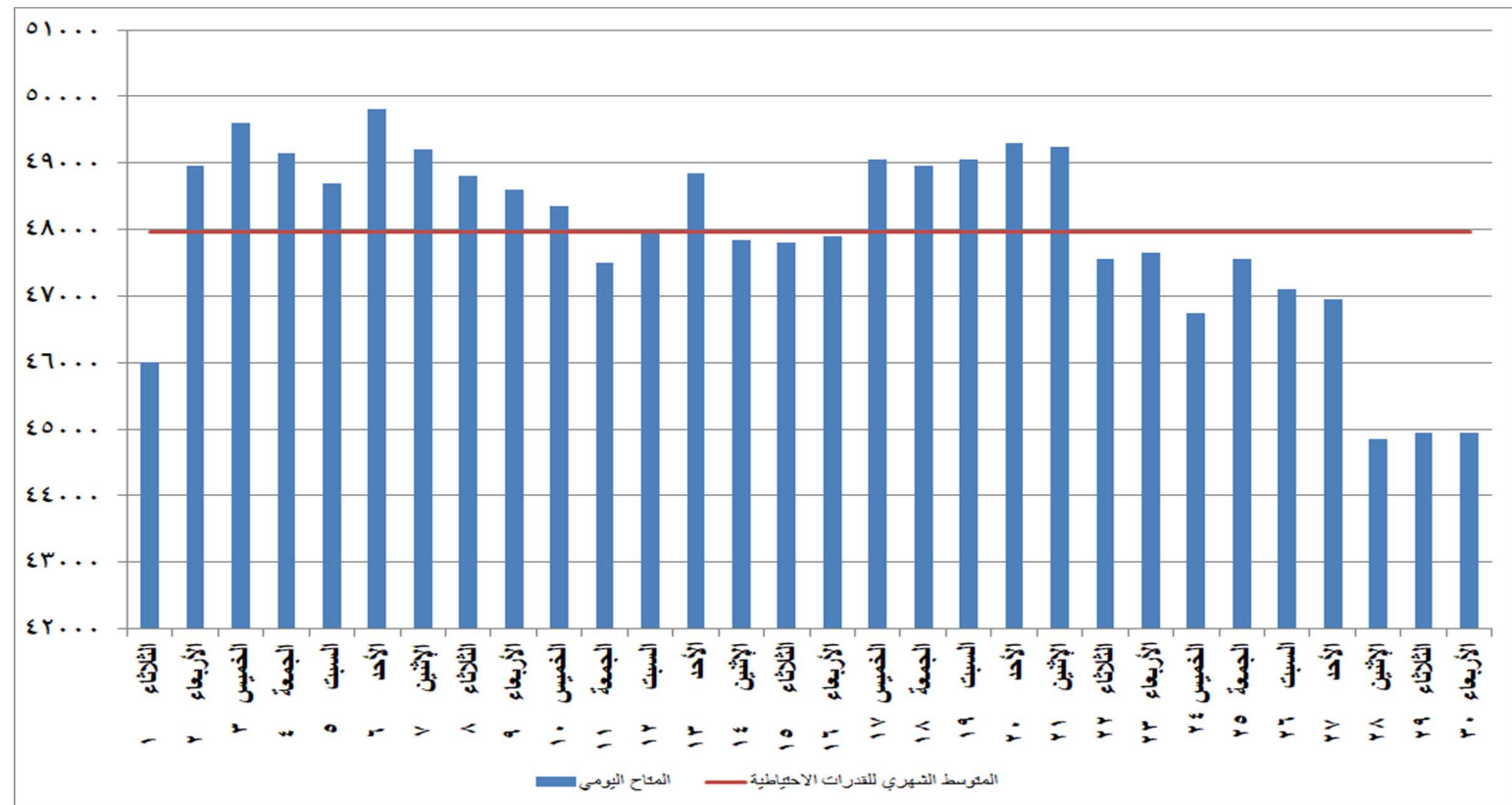
شكل (٢٧) القدرات المتاحة يوميا والمتوسط الشهري للقدرات الاحتياطية خلال شهر يونيو ٢٠٢١
