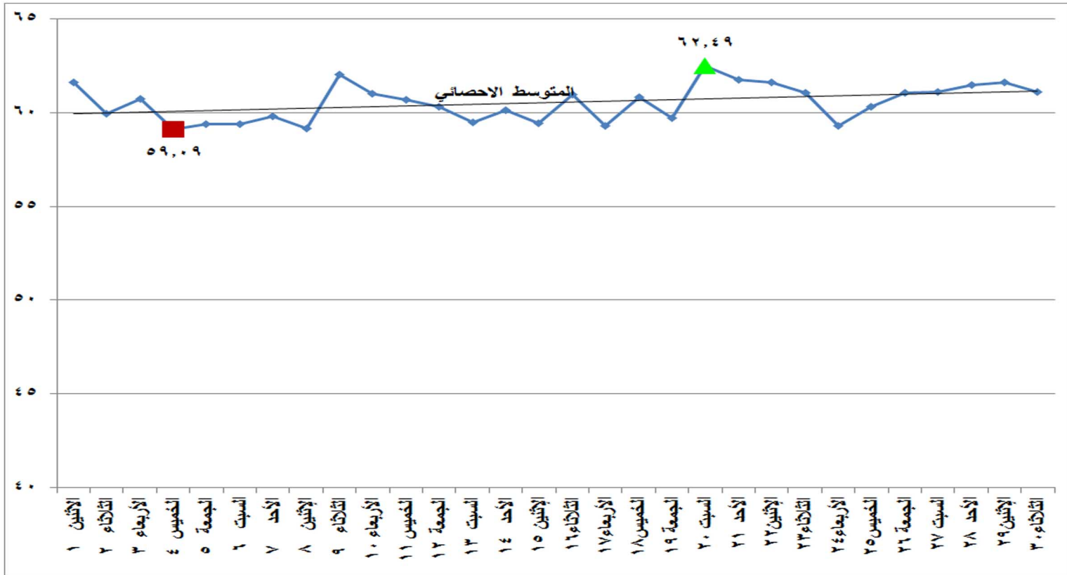
شكل (٢٣) الطاقة الكهربائية المنتجة من المصادر المائية خلال شهر يونيو ٢٠٢١
