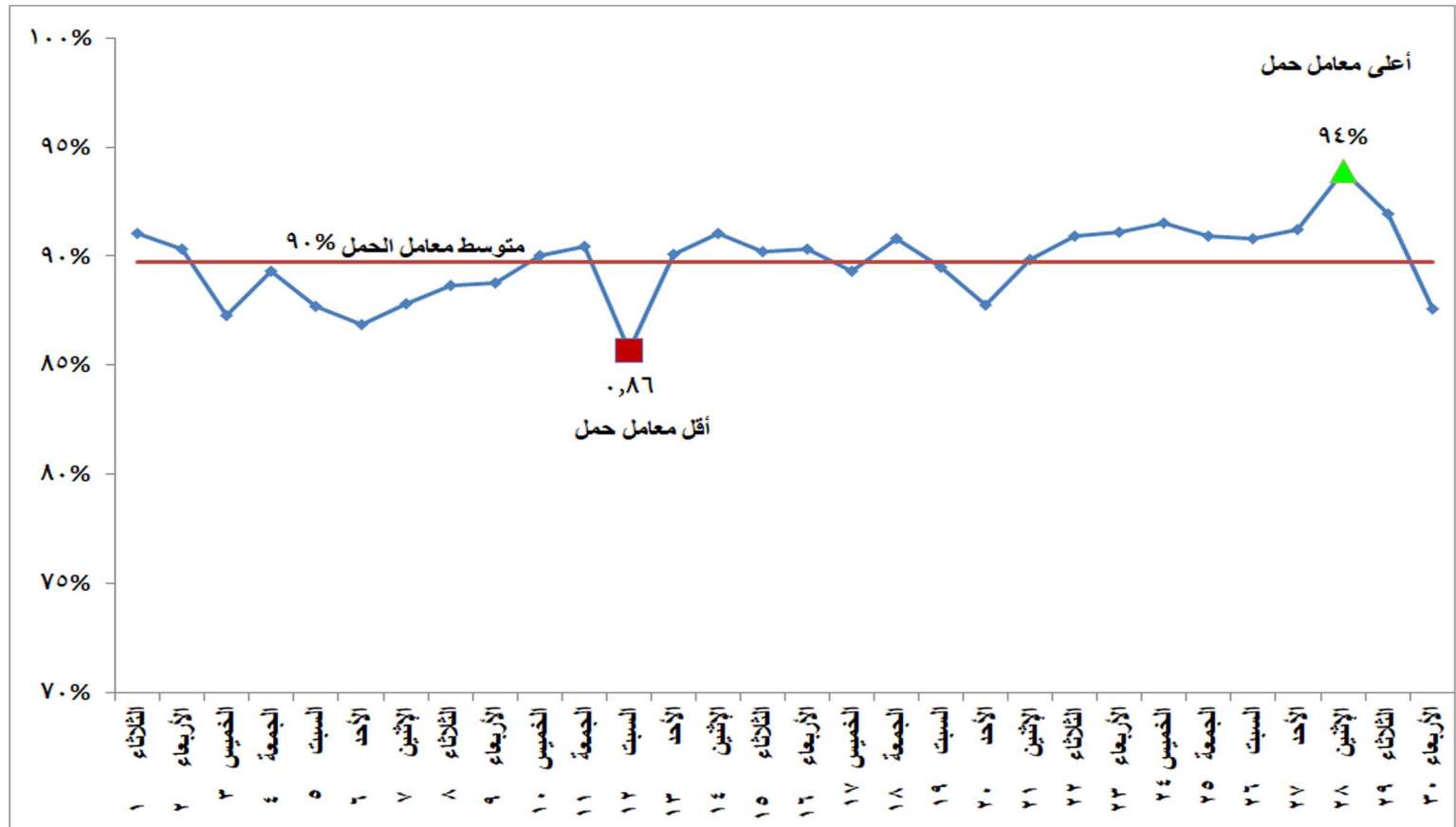
شكل (١٢) إجمالي معامل الحمل لوحدات الانتاج خلال شهر يونيو ٢٠٢١
