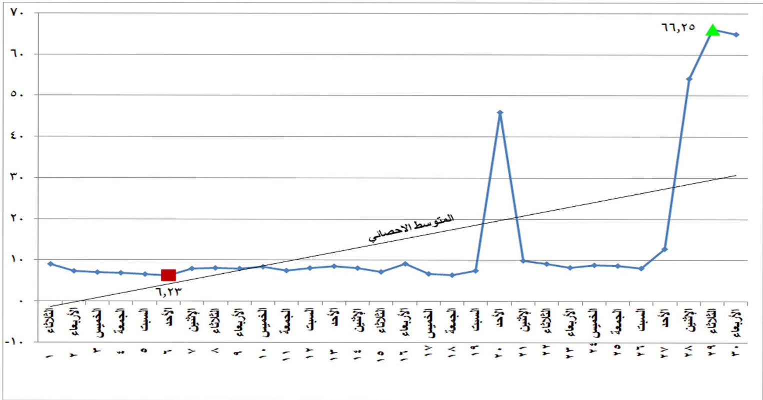
شكل (١٩) الطاقة الكهربائية المنتجة من المازوت خلال شهر يونيو ٢٠٢١
