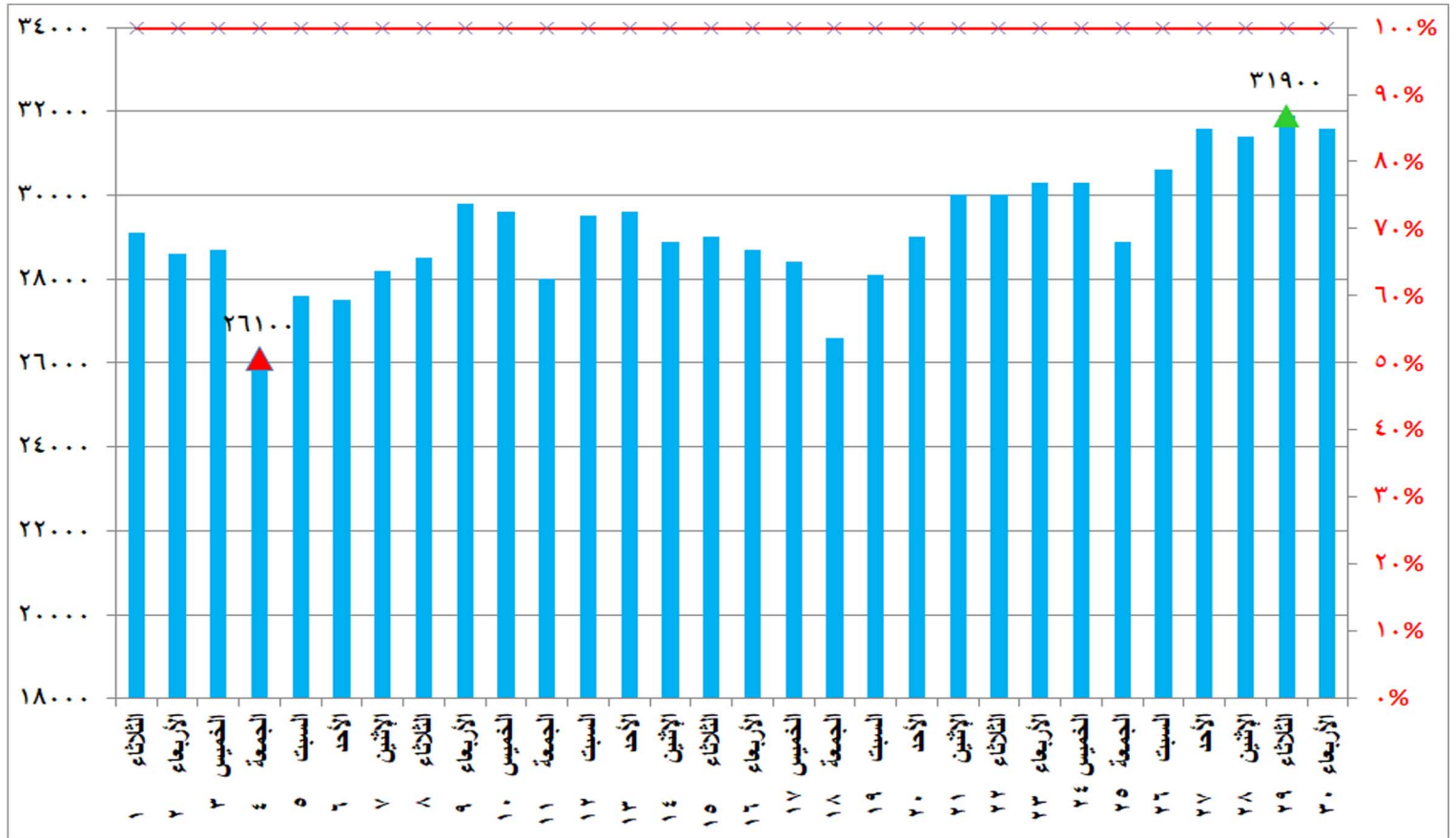
شكل (٥) قدرات الانتاج المتاحة ونسبتها للحمل الأقصى خلال شهر يونيو ٢٠٢١
