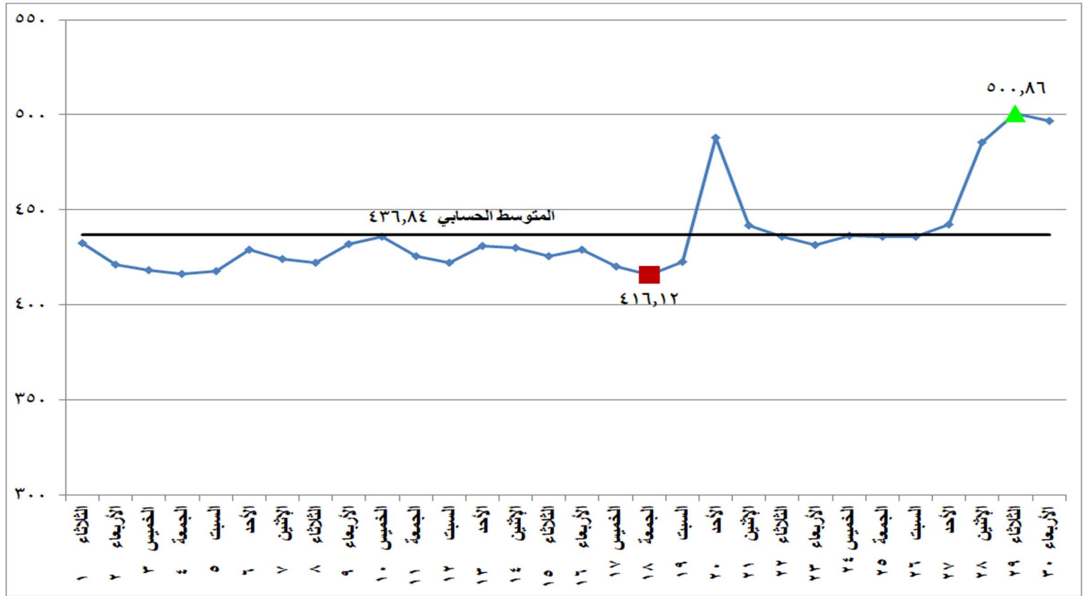
شكل (١٥) إجمالي الطاقة الكهربائية المنتجة من كل المصادر الأولية خلال شهر يونيو ٢٠٢١
